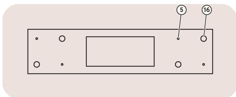
Afbeelding 7: Boven aanzicht van de gaten in de vloerplaat
