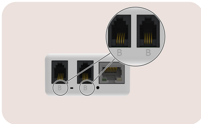
Afbeelding 14: aanzicht op B-poorten van de Smappee Connect
